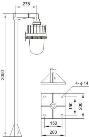
法兰式(f1) Bend type
