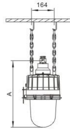
吊链式(D) Hanging chain type
