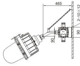
壁式(B1) Bracket type 30°
