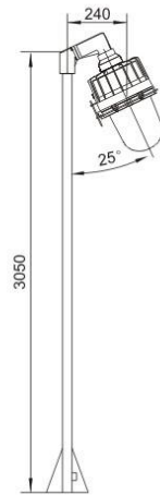
法兰式(f2) Bend type
