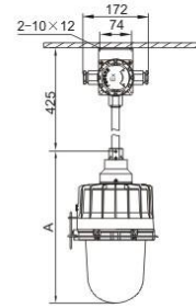
吊杆式(G) Pendant type
