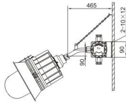
壁式(B1) Bracket type 30°
